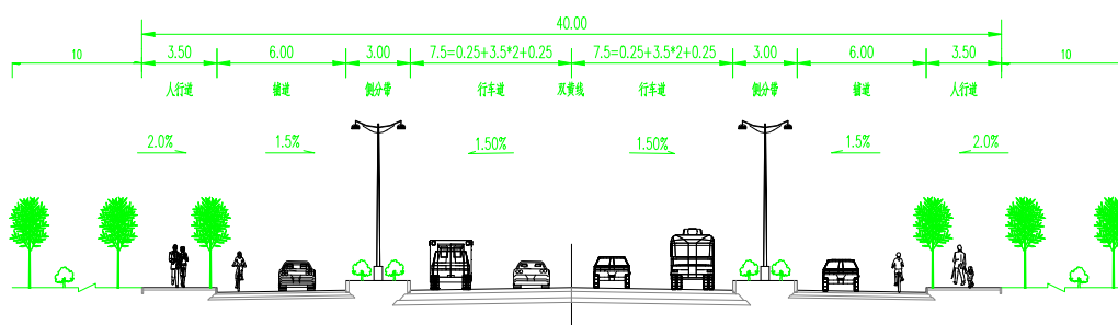
道路典型横断面图 (40m) 工业园1号路
